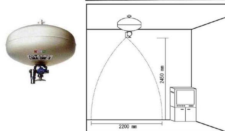
図4. 消火具の例②
